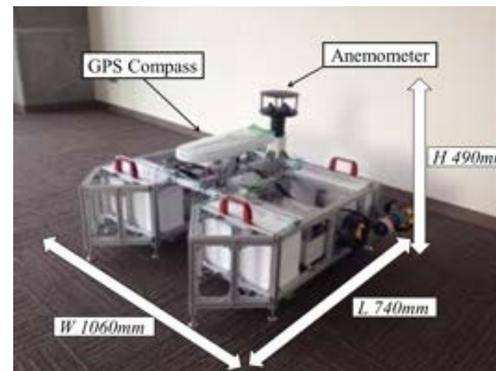
No.2 水上ロボット
